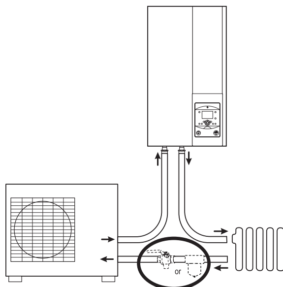
Abb. 7 - Installation des Filterventils
