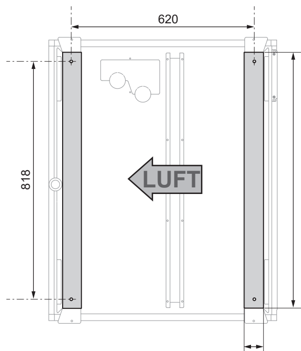
Abb. 4 - Abmessungen der Halterungen der Außeneinheit
