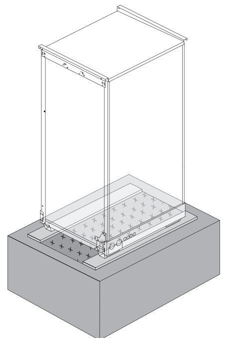
Abb. 5 - Sockel der Außeneinheit
