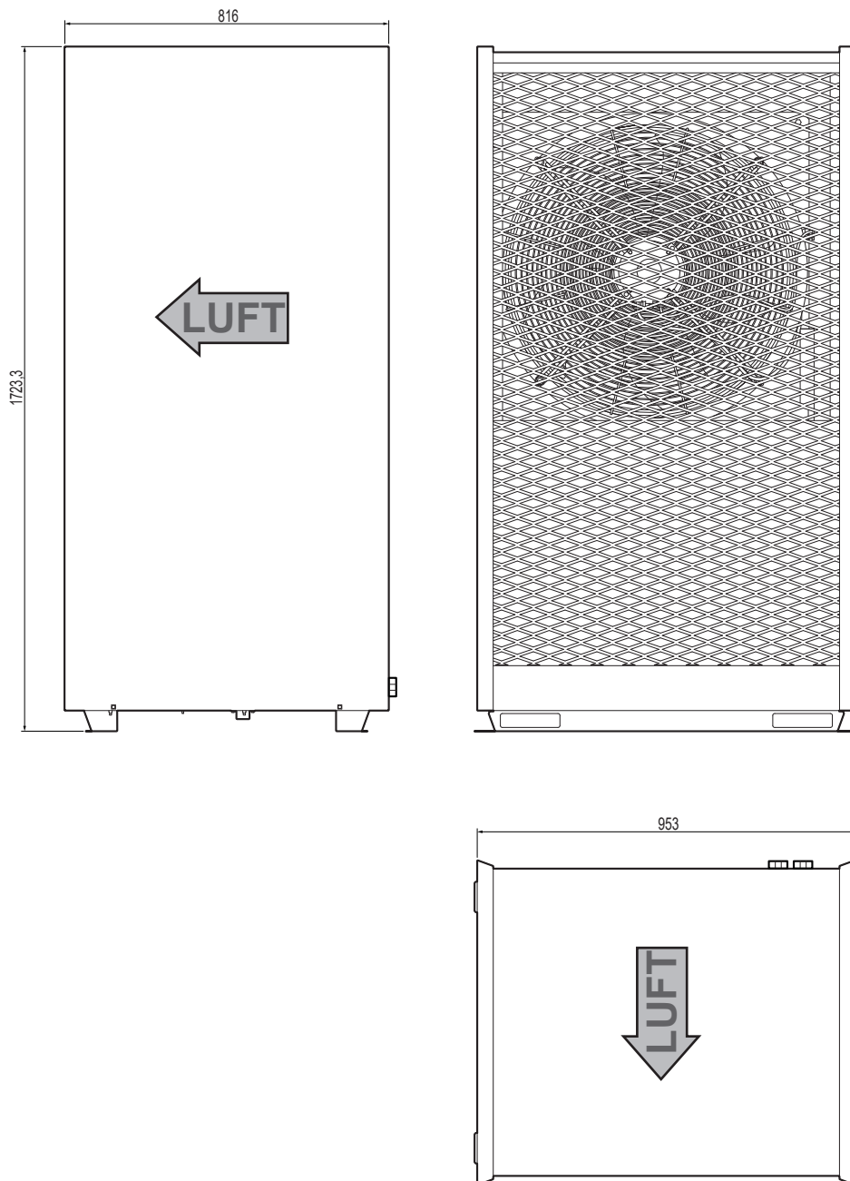
Abb. 1 - Abmessungen (in mm)
