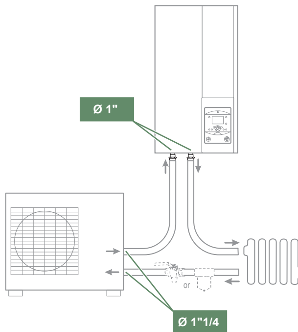
Abb. 6 - Durchmesser der Anschlussstücke der Rohrleitungen
