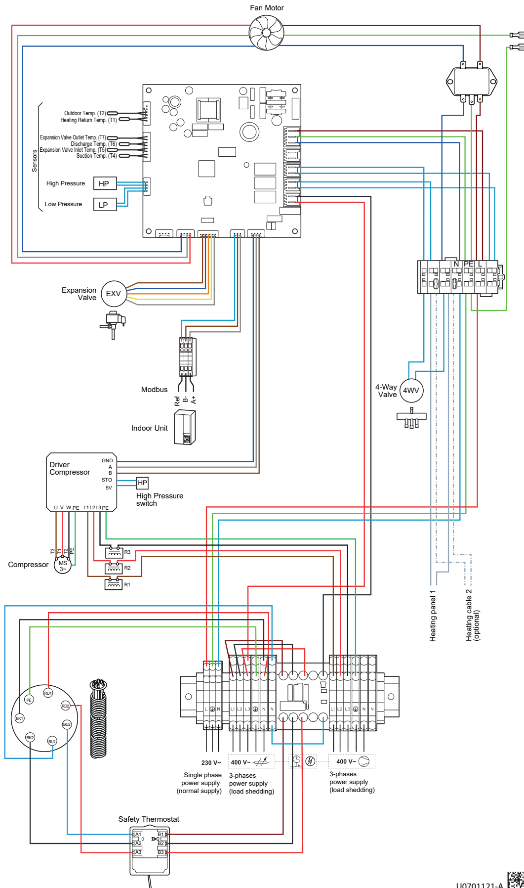
Abb. 9 - Stromlaufplan Außereinheit Modell LWPM 11 OUTDOOR
