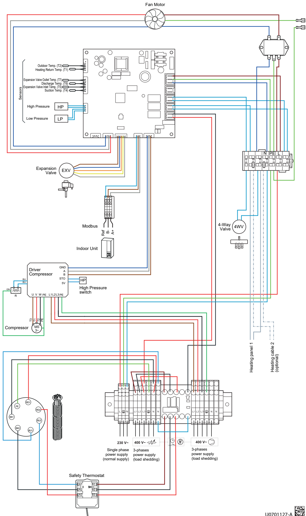
Abb. 10 - Stromlaufplan Außeneinheit Modell LWPM 14 OUTDOOR
