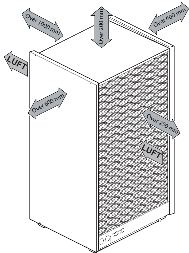
Abb. 3 - Installationsmindestfreiräume um die Außeneinheit
